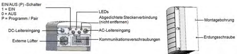
Abbildung 6: Schnittstellen auf der Unterseite und an der Seite der Primäreinheit
